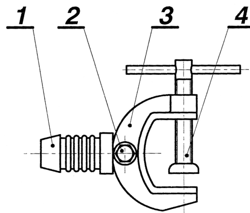
Poz. 1 Osłona gumowa Poz. 2 Wkręt specjalny Poz. Obejma Poz. Śruba specjalna
